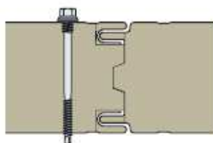
KS1000 FR Verticale aansluiting
