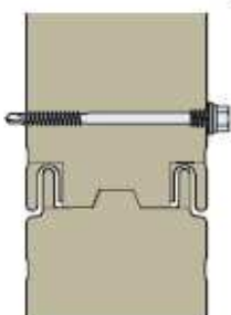
KS1000 FR Horizontale aansluiting
